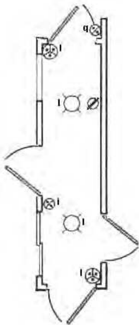
Figura 4.9. Pasillo dos, área AO10.
