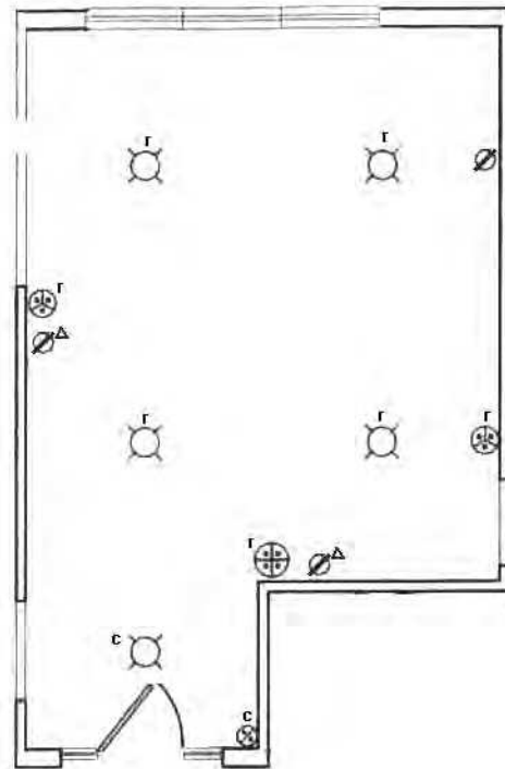
Figura 4.13. Sala de descanso, área AO14.
