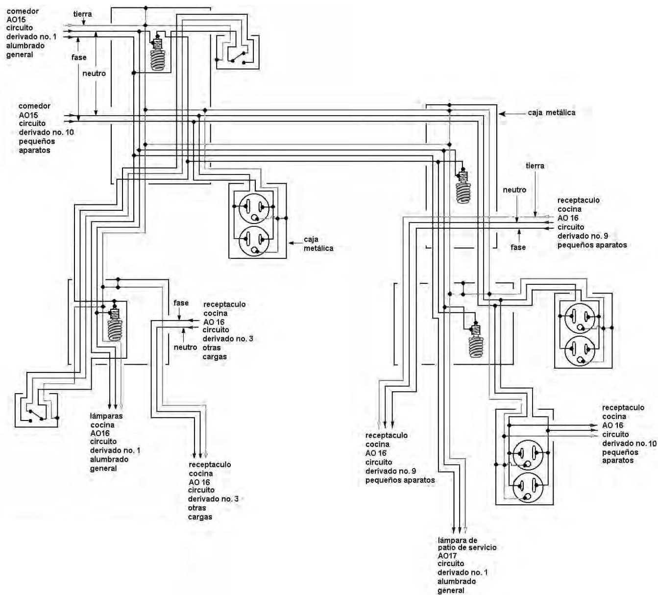
Figura 4.56. Comedor, área AO15. Circuito de alambrado
