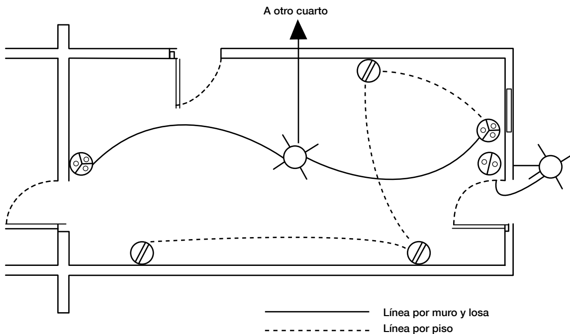
Planta simplificada de un cuarto de una casa habitación, mostrando posibles trayectorias de tubo (conduit) para alambrado a las salidas.
