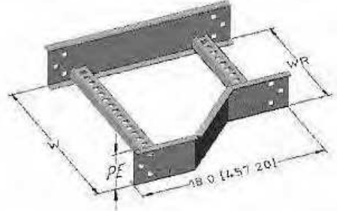
Charola con Reducción Lateral
