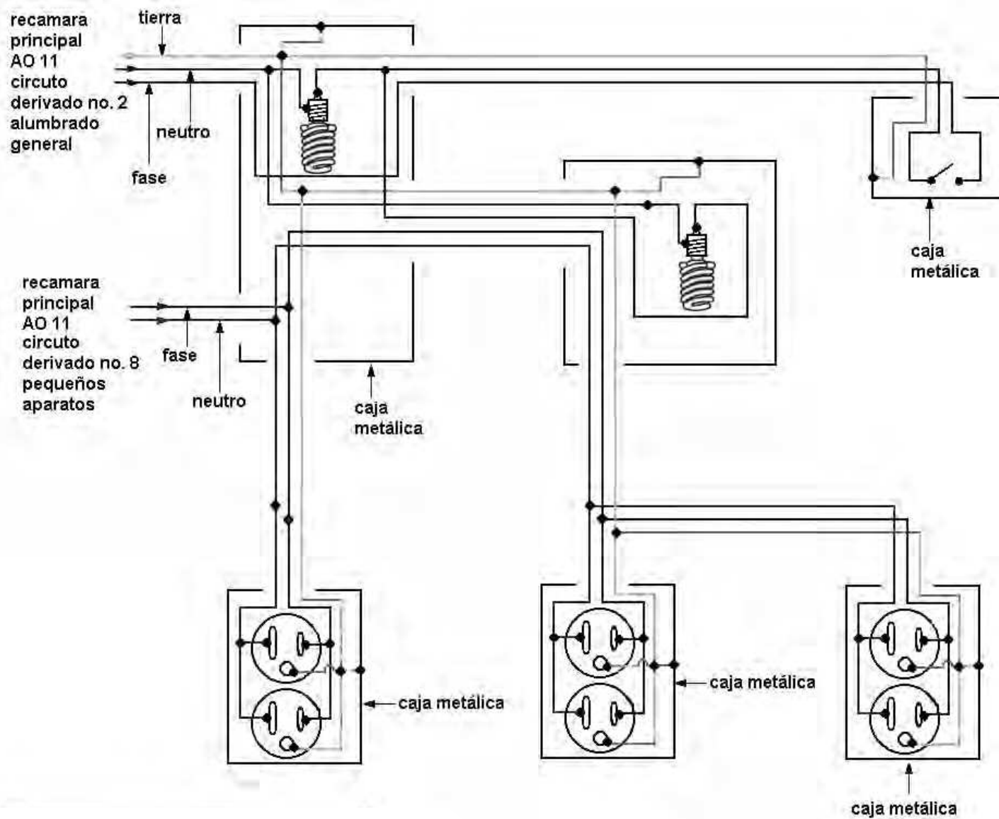
Figura 4.48. Recámara principal, área AO11. Circuito de alambado
