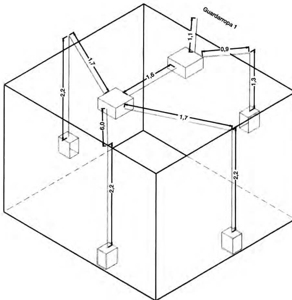
Figura 4.42. Vista en isométrico de tuberías y cajas de conexión. Recámara 1, área AO7.
