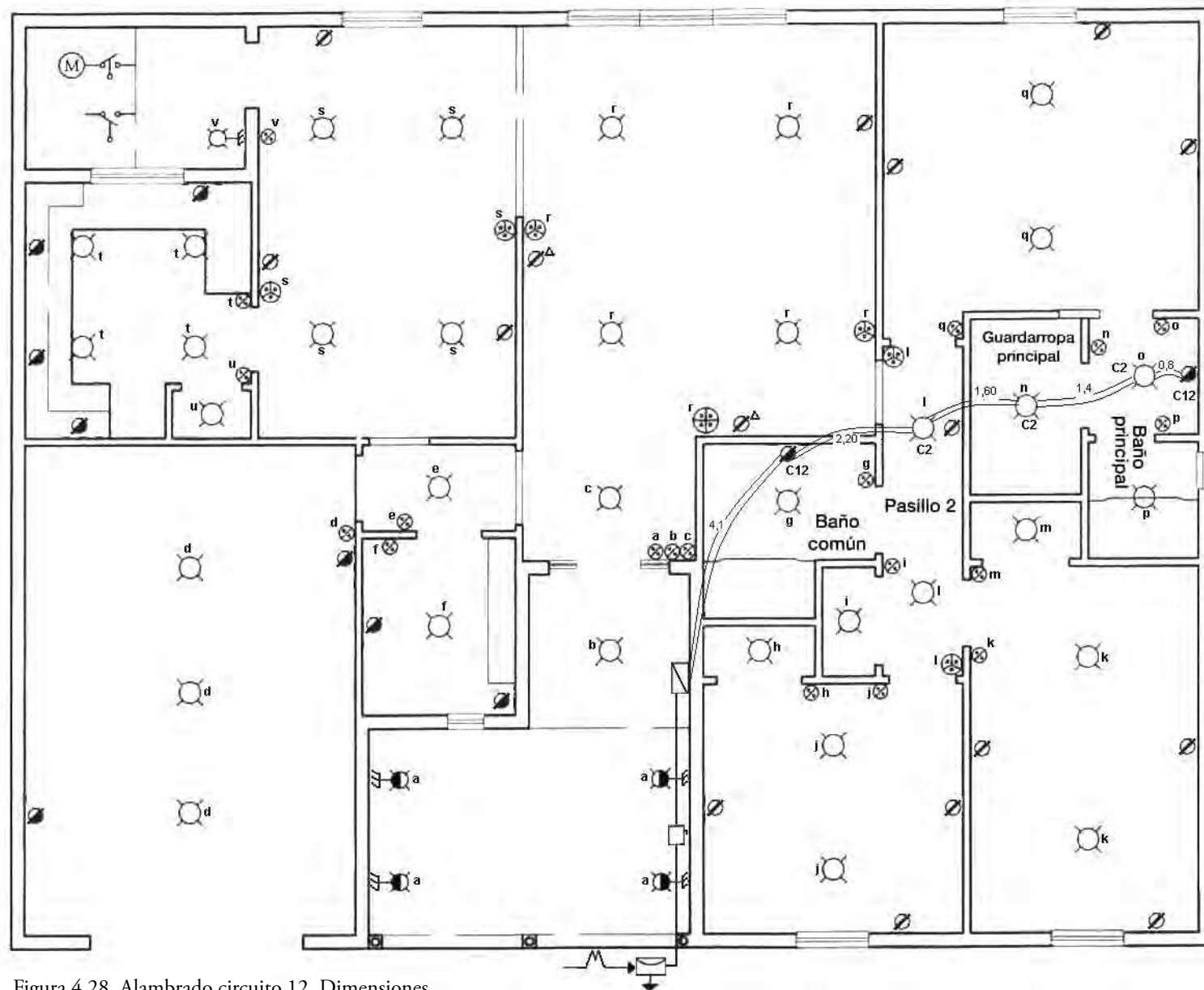
Figura 4.28. Alambrado circuito 12. Dimensiones.
