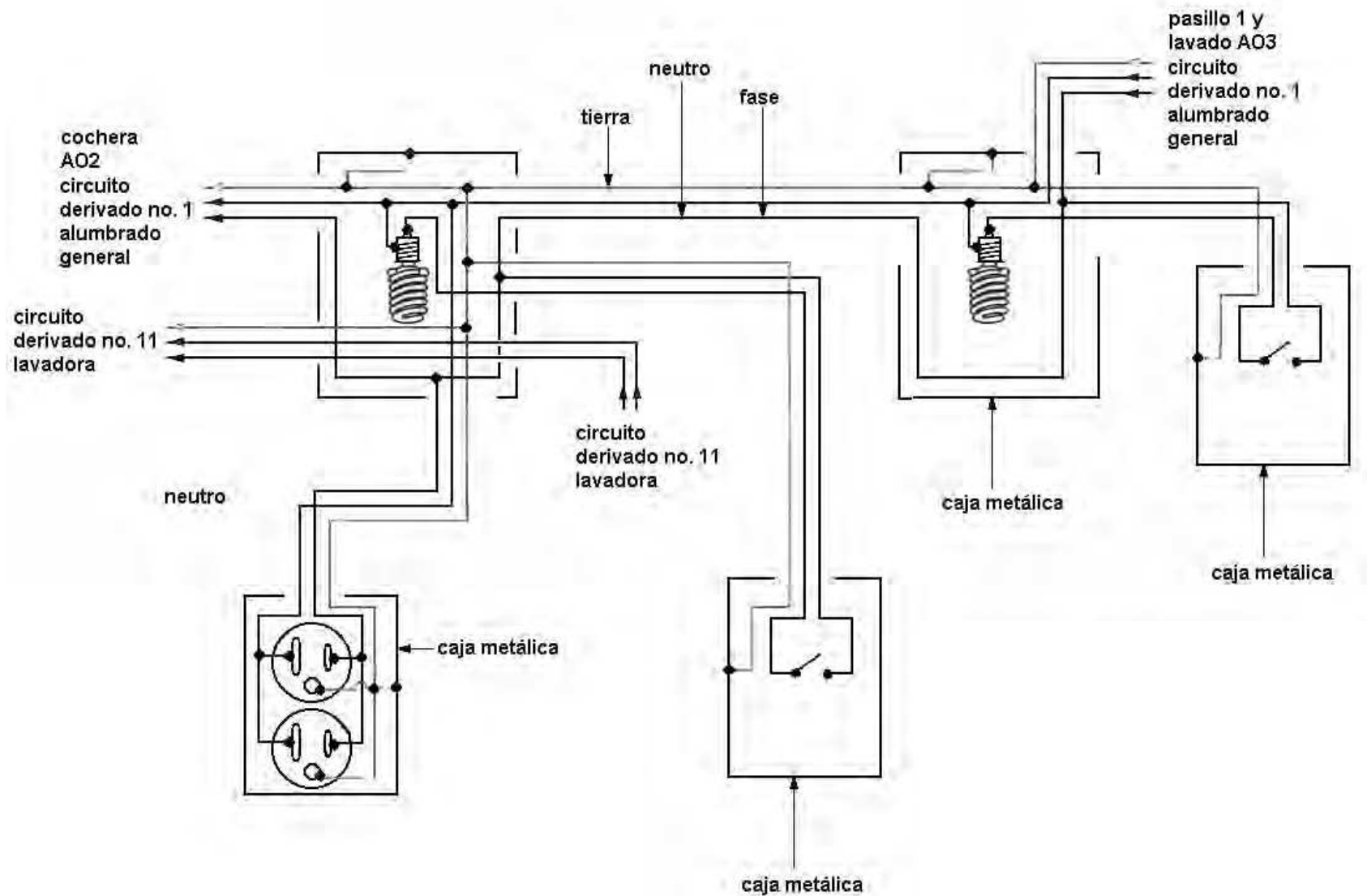
Figura 4.35. Pasillo 1 y cuarto de lavado, área AO3. Circuito de alambrado.
