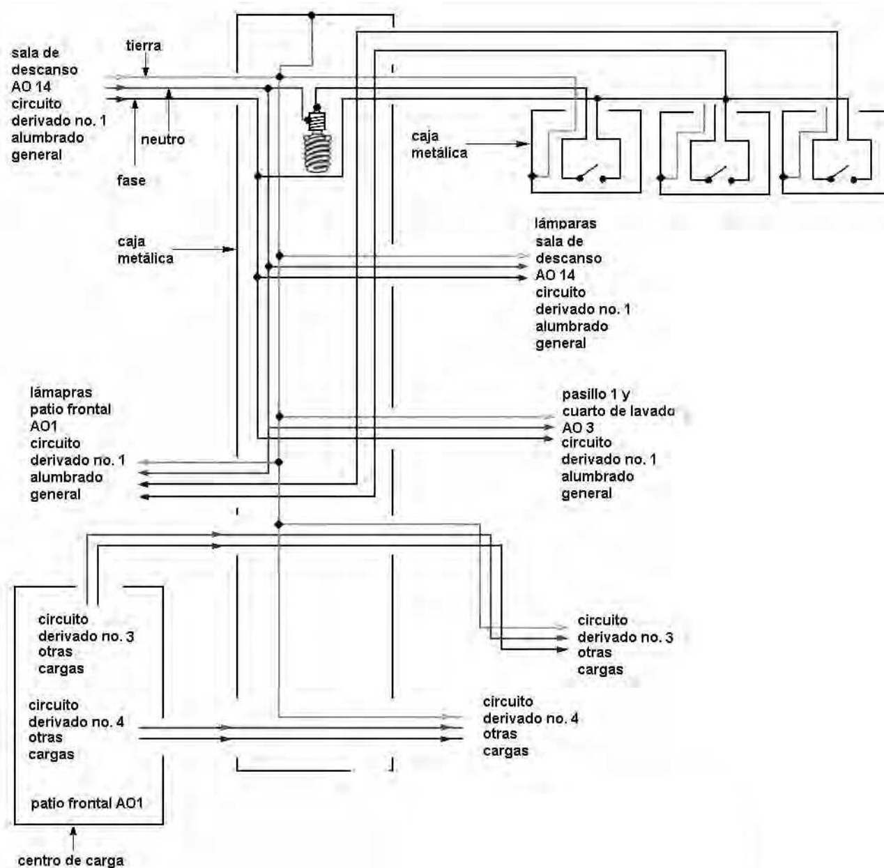
Figura 4.53. Sala de descanso AO14. Circuito de alumbrado No. 1
