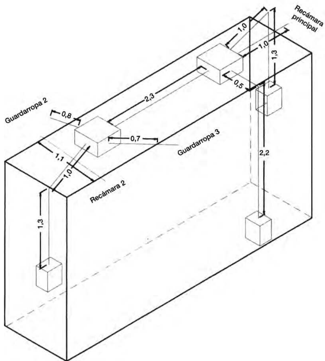
Figura 4.47. Vista en isométrico de tuberías y cajas de conexión. Pasillo 2, área AO10.
