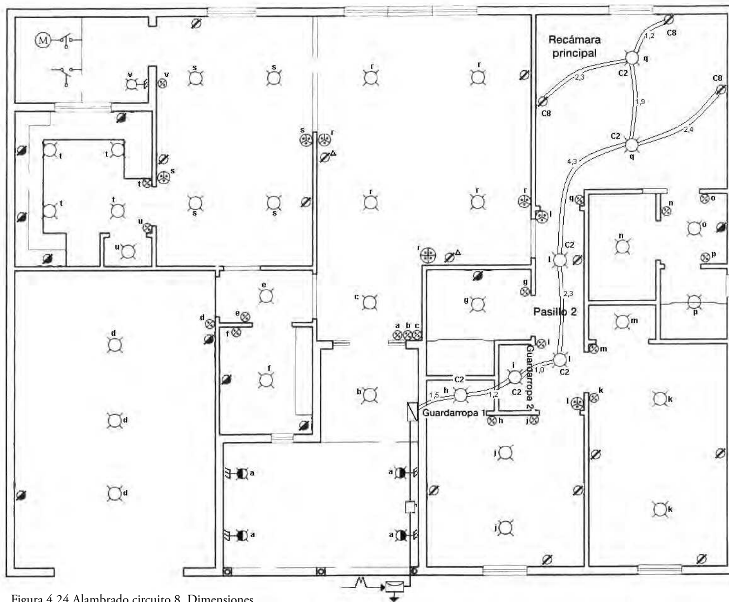
Figura 4.24 Alambrado circuito 8. Dimensiones.
