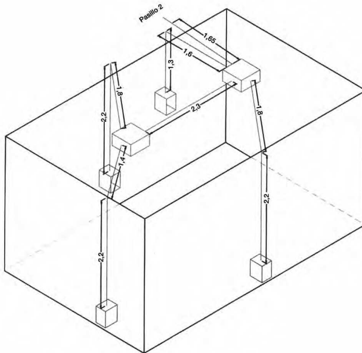
Figura 4.44. Vista en isométrico de tuberías y cajas de conexión. Recámara 2, área AO8.
