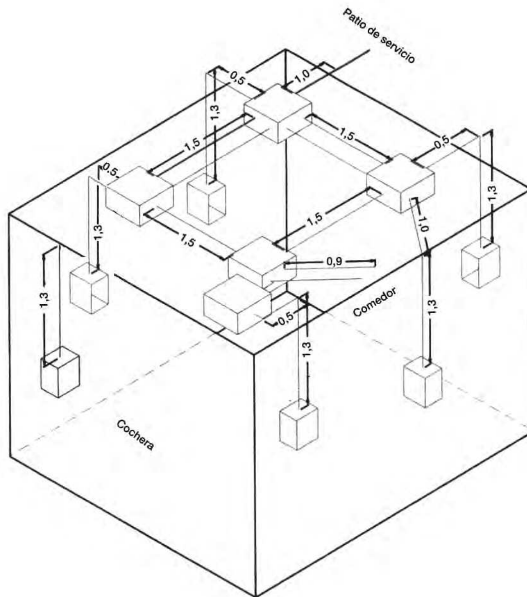
Figura 4.59. Vista en isométrico de tuberías y cajas de conexión. Cocina, área AO16.
