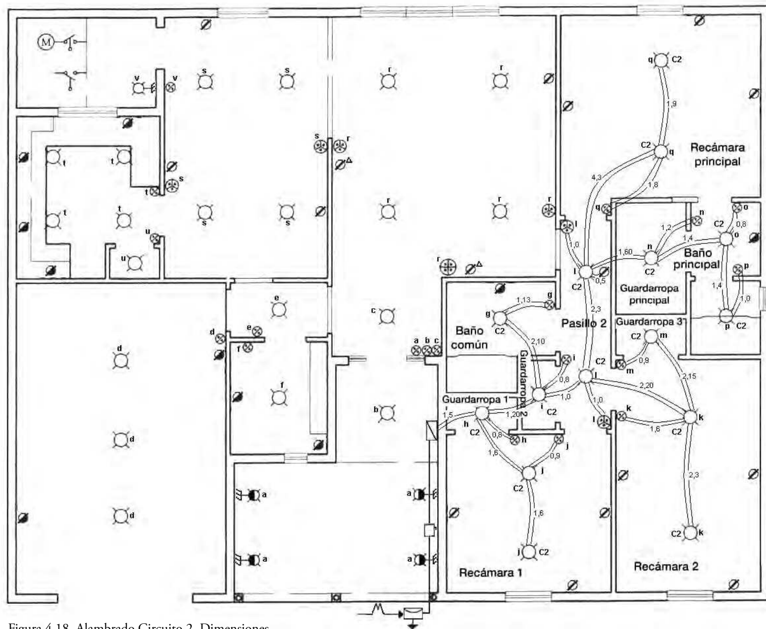
Figura 4.18. Alambrado Circuito 2. Dimensiones.
