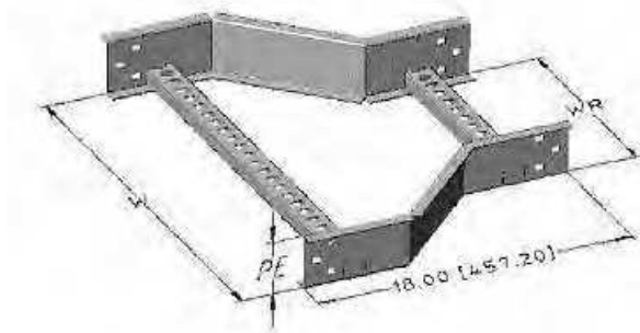
Charola con Reducción Recta (HRR)
