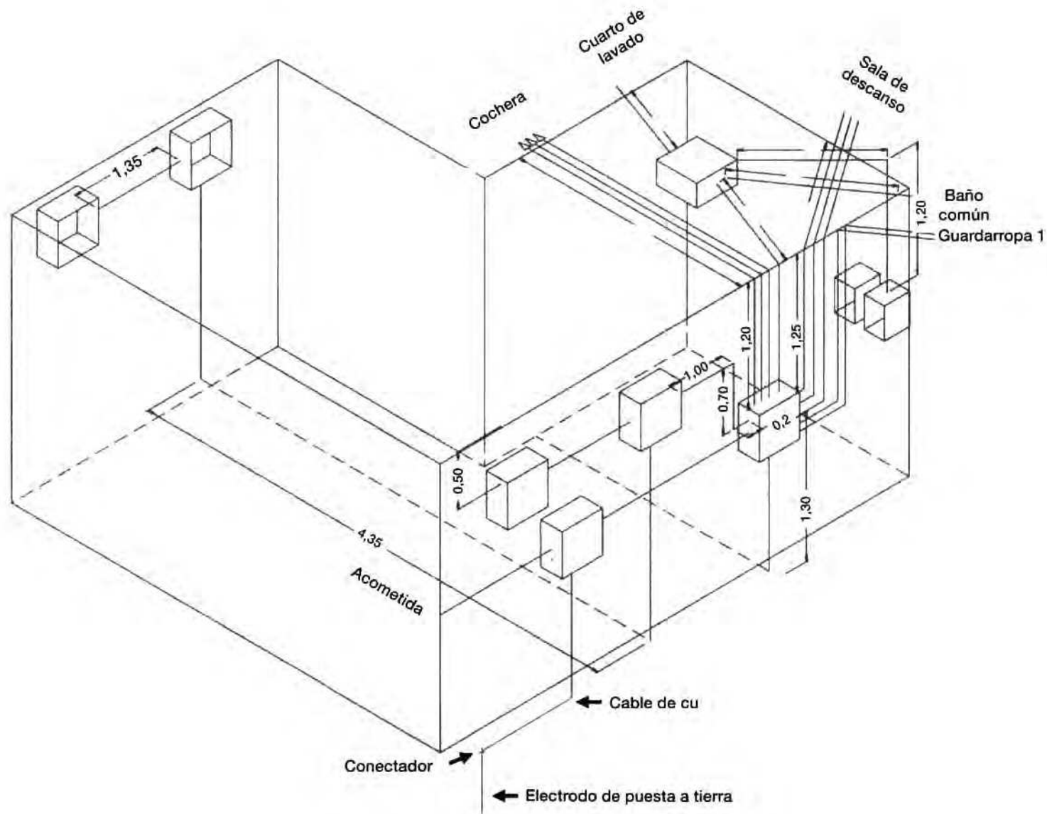
Figura 4.32. Vista en isométrico de tuberías y cajas de conexión. Patio frontal, área AO1.
