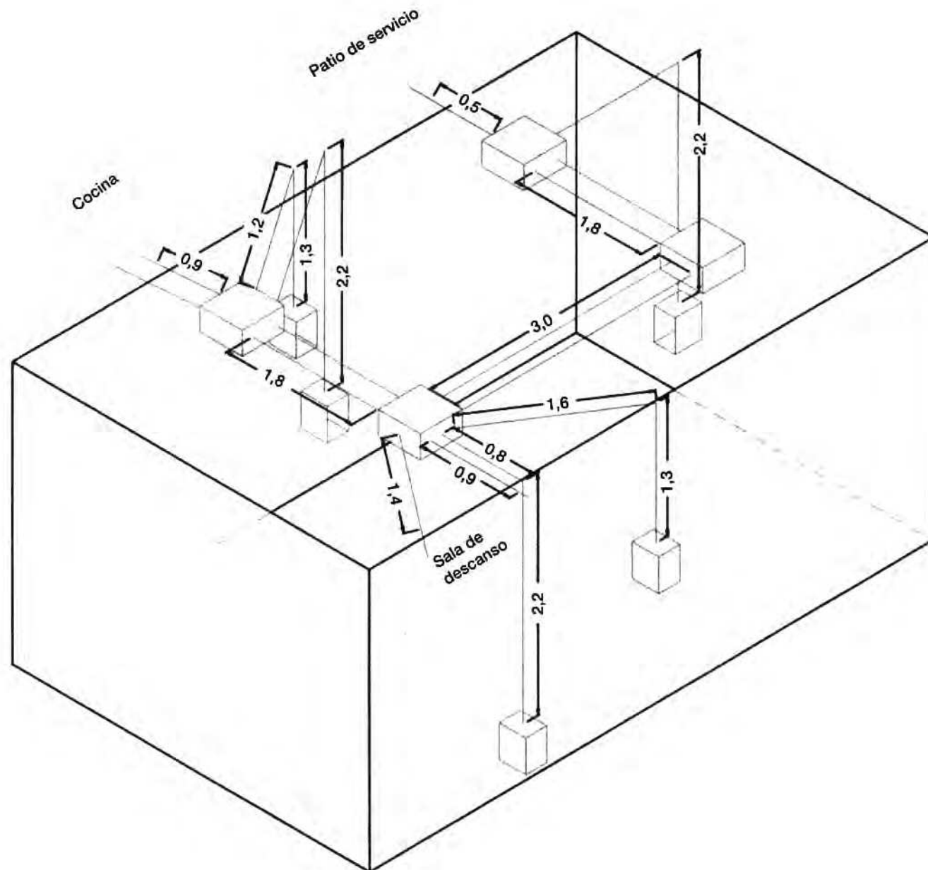
Figura 4.57. Vista en isométrico de tuberías y cajas de conexión. Comedor, área AO15.
