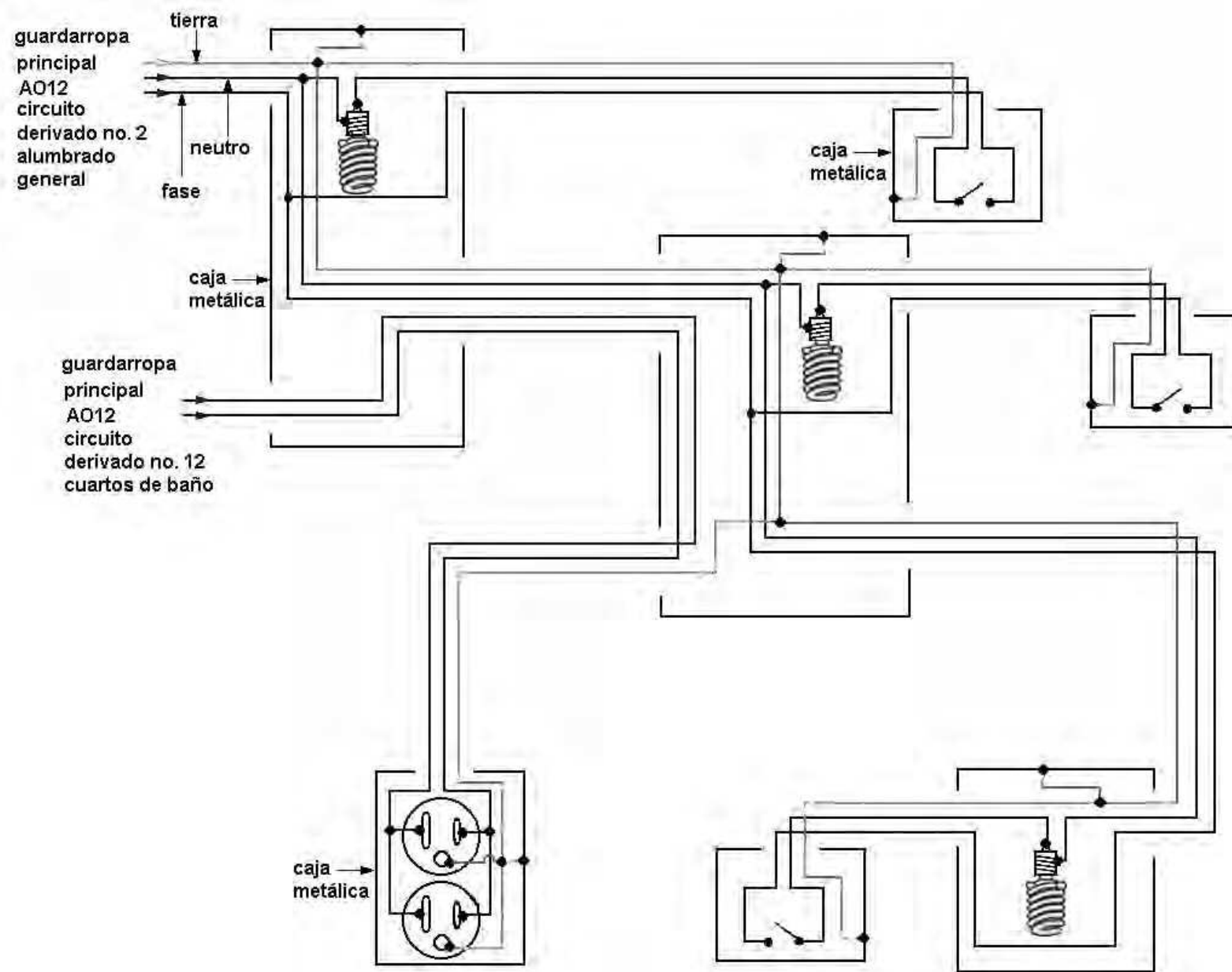
Figura 4.50. Guardarropa principal, área A012 y baño principal, área AO13. Circuito de alambrado.
