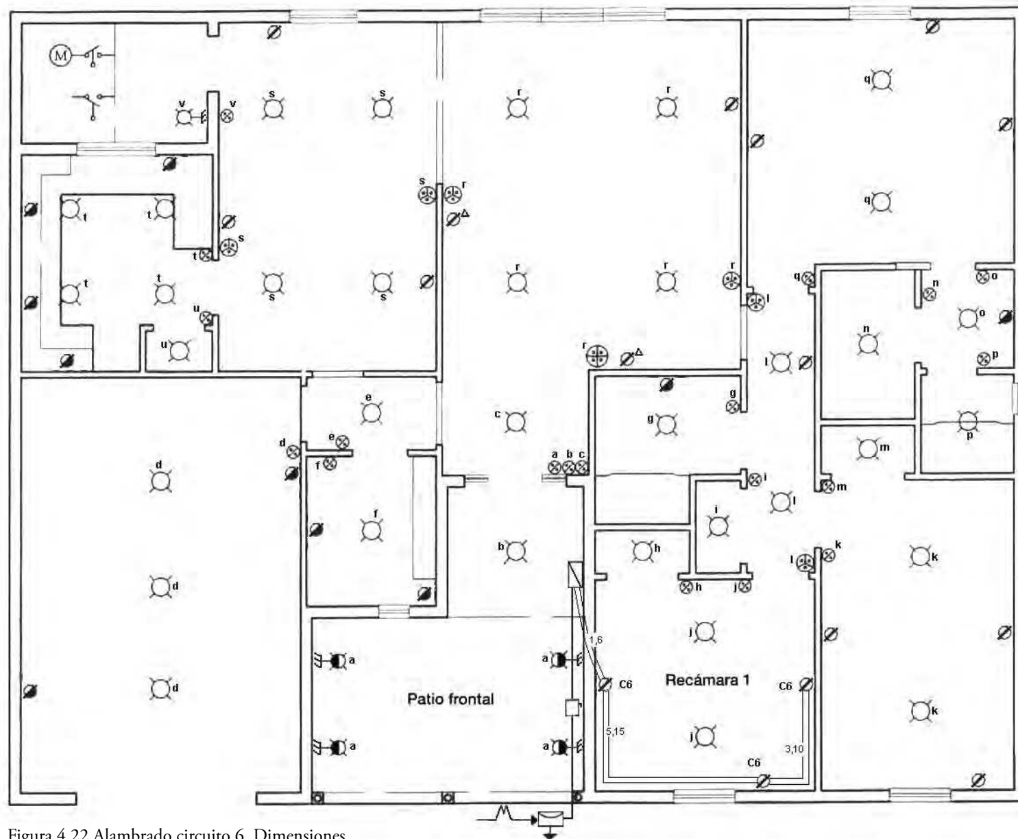
Figura 4.22 Alambrado circuito 6. Dimensiones.
