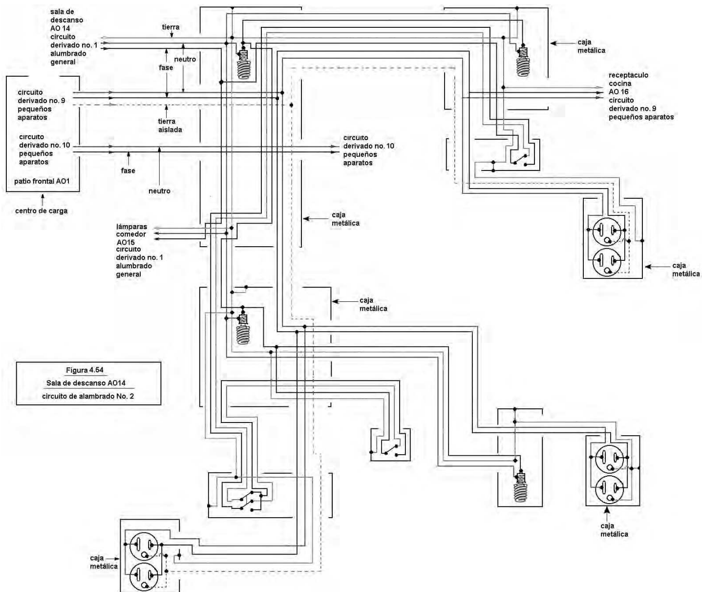
Figura 4.54. Sala de descanso AO14. Circuito de alambrado No. 2
