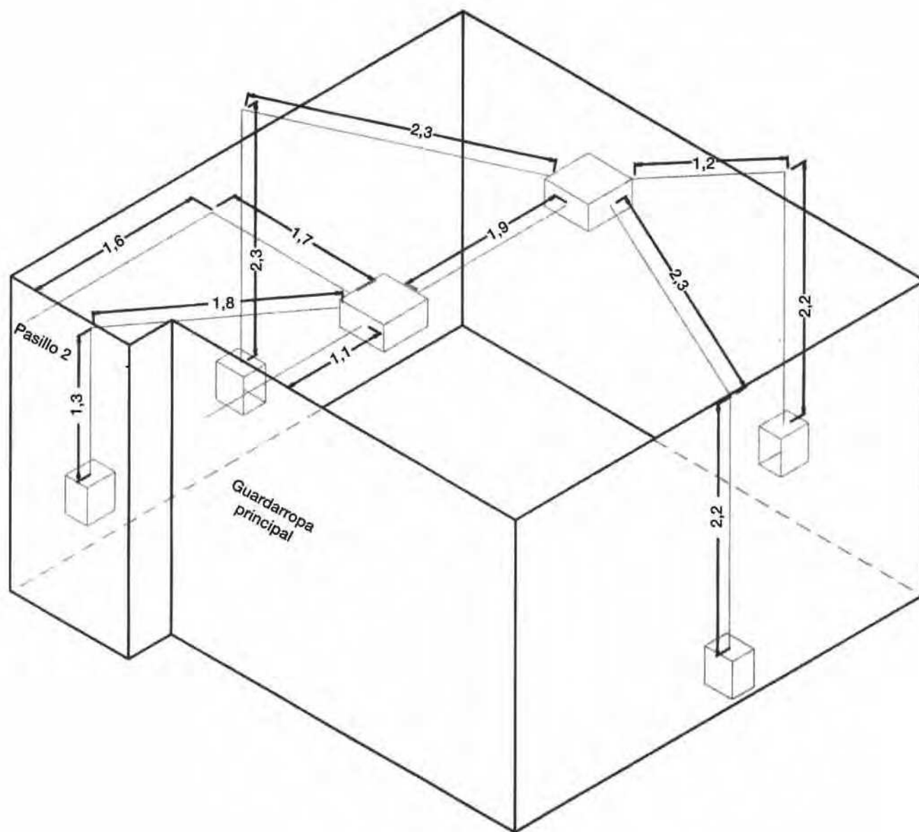
Figura 4.49. Vista en isométrico de tuberías y cajas de conexión. Recámara principal, área AO11.
