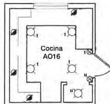
Figura 4.15. Cocina, área AO16.
