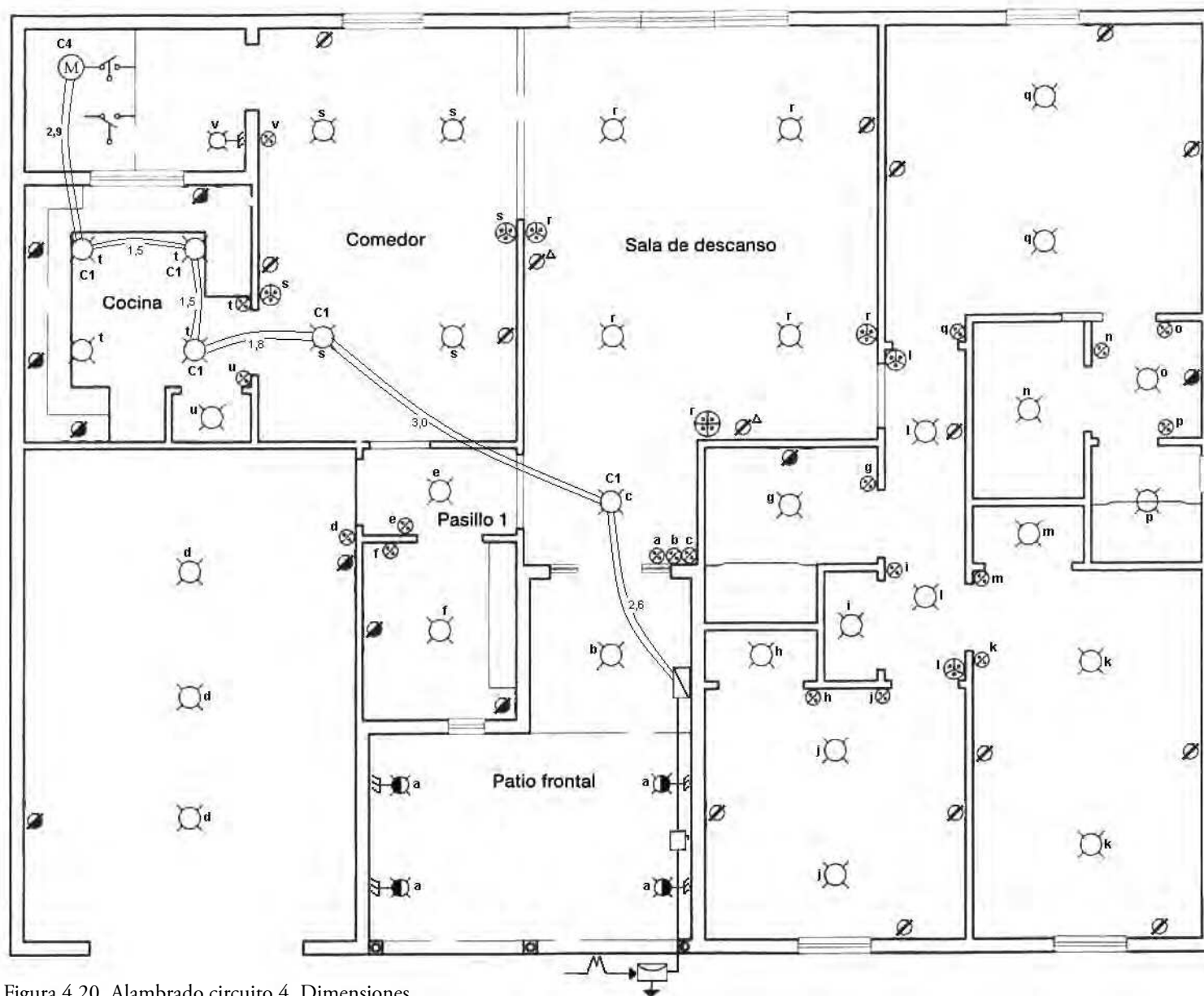
Figura 4.20. Alambrado circuito 4. Dimensiones.
