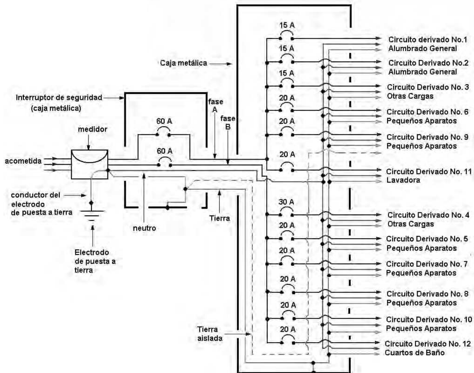
Figura 4.30. Patio frontal, área AO1. Circuito para acometida, alimentador y tablero.
