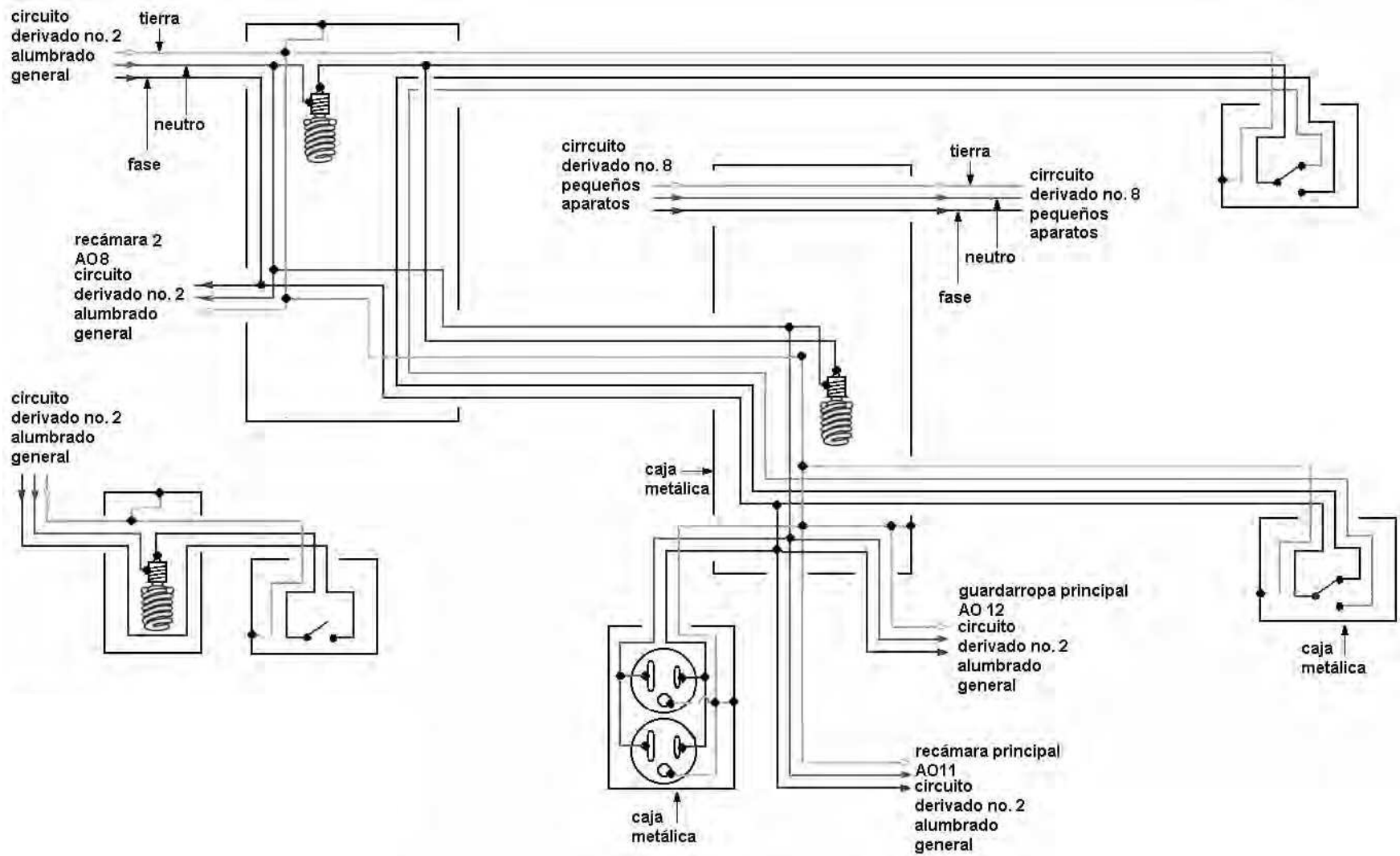
Figura 4.45. Pasillo 2, área AO10 y guardarropa 3, área AO9. Circuito de alambado.
