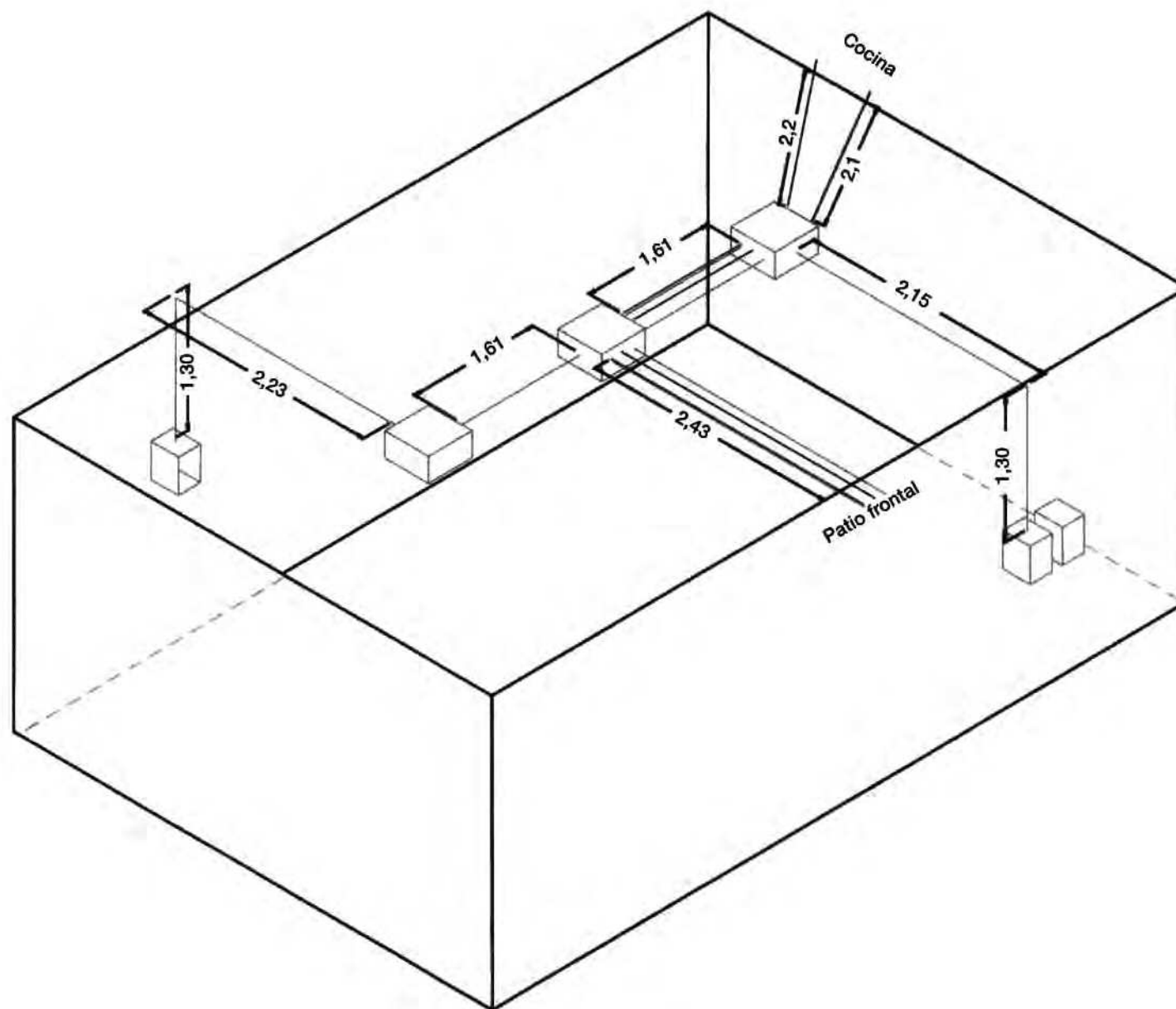
Figura 4.34. Vista en isométrico de tuberías y cajas de conexión. Cochera, área AO2.
