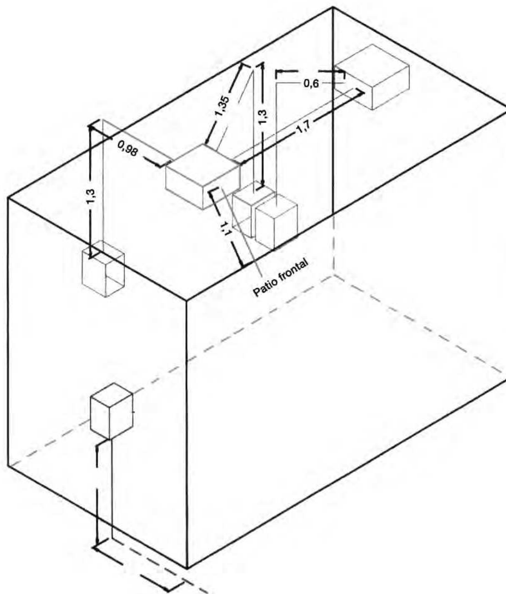
Figura 4.36. Vista en isométrico de tuberías y cajas de conexión. Pasillo 1 y cuarto de lavado, área AO3.
